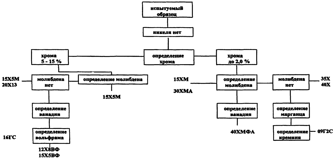
Рисунок 2 – Схема очередности определения для разбавки низколегированных и легированных сталей
